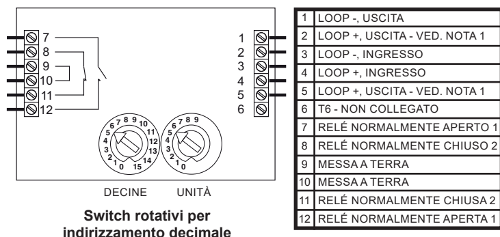
Figure 2: Cablaggio del modulo
