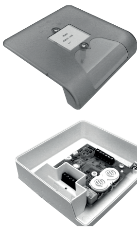
Abbildung 1a: M201E-240 (-KO) Steuermodul zur aP-Montage mit Relais für Netzspannung
