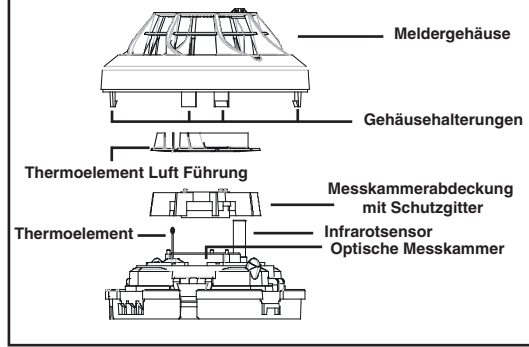
Abbildung 2: Reinigung des Melders
