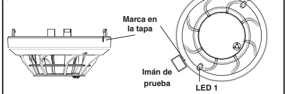
Figura 3: Posición del imán de prueba
