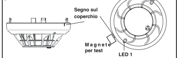
Figura 3: Posizione del magnete per il test
