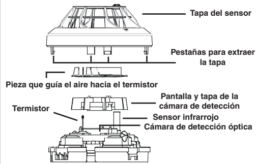
Figura 2: Limpieza del sensor
