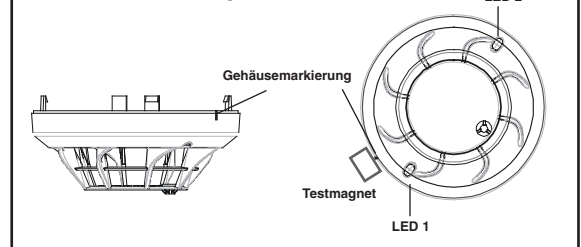
Abb. 3: Position des Testmagneten
